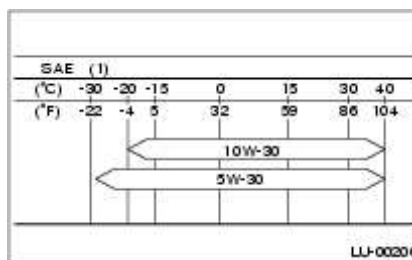
(1) SAE粘度指数および適用温度
