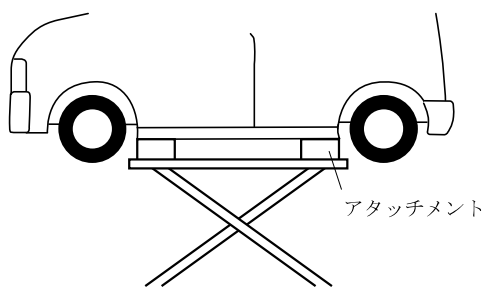
ボードオンリフト支持例
